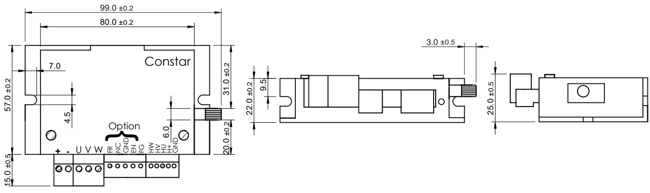
M 1:2 型号 / Model S17-112503H-FR/S17-114820H-FR
